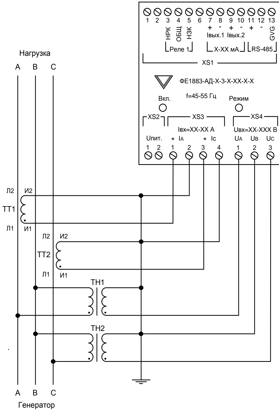
Рисунок Д.3 – Схема подключения преобразователя по трехпроводной схеме с помощью двух трансформаторов тока и двух трансформаторов напряжения
