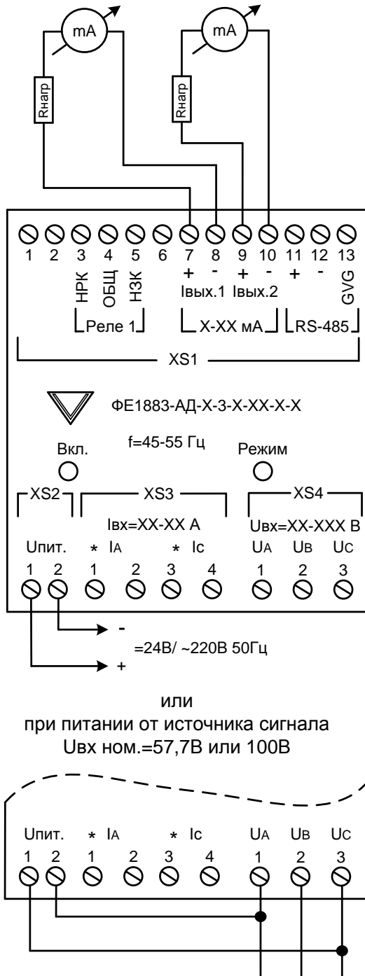
Рисунок Д.8 – Схема подключения цепей питания и унифицированного выхода постоянного тока для преобразователей по трехпроводной схеме.
