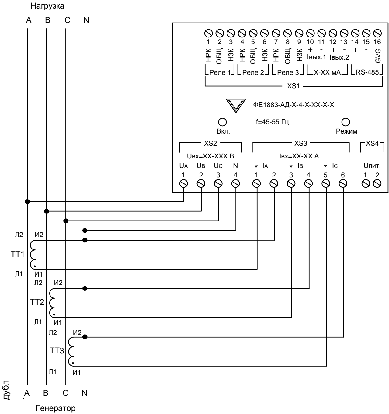
Рисунок Д.6 – Схема подключения преобразователя по четырехпроводной схеме с помощью трех трансформаторов тока
