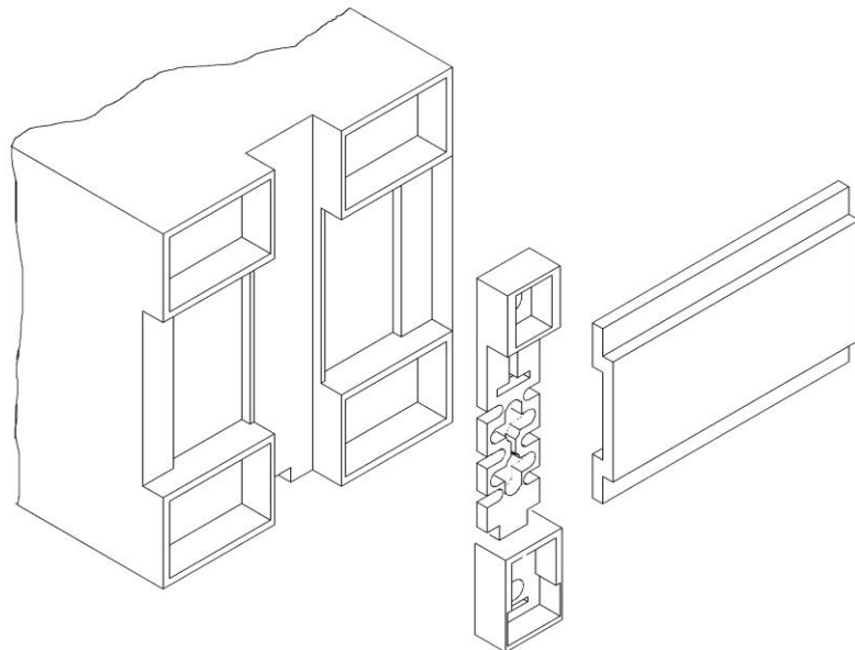
Рисунок В.2 – Монтаж преобразователя на DIN-рейку
