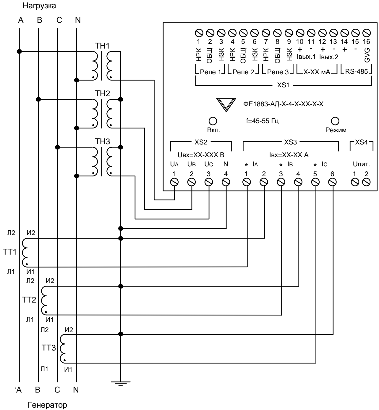
Рисунок Д.5 – Схема подключения преобразователя по четырехпроводной схеме с помощью трех трансформаторов тока и трех трансформаторов напряжения
