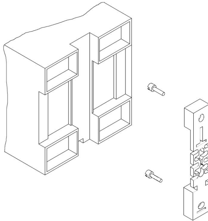
Рисунок В.1 – Монтаж преобразователя на щит или на панель
