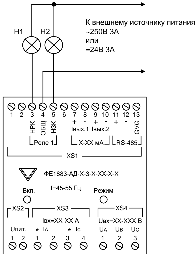
Рисунок Д.10 – Схема подключения цепей внешней сигнализации и управления к преобразователю по трехпроводной схеме
