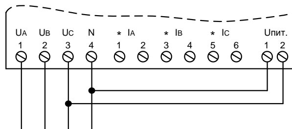
Рисунок Д.9 – Схема подключения цепей питания и унифицированного выхода постоянного тока для преобразователей по четырехпроводной схеме
